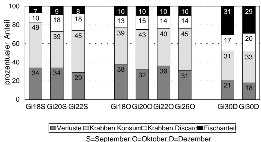
Abb. 1: Anteilige Zusammensetzung des Gesamtfanges bei verschiedenen Sortiergittereinsätzen bei 9-m-Garnelenbaumkurren (Gi18S (Gi=Gitter, 18=lichte Weite in mm zwischen den Gitterstäben, S=September)
