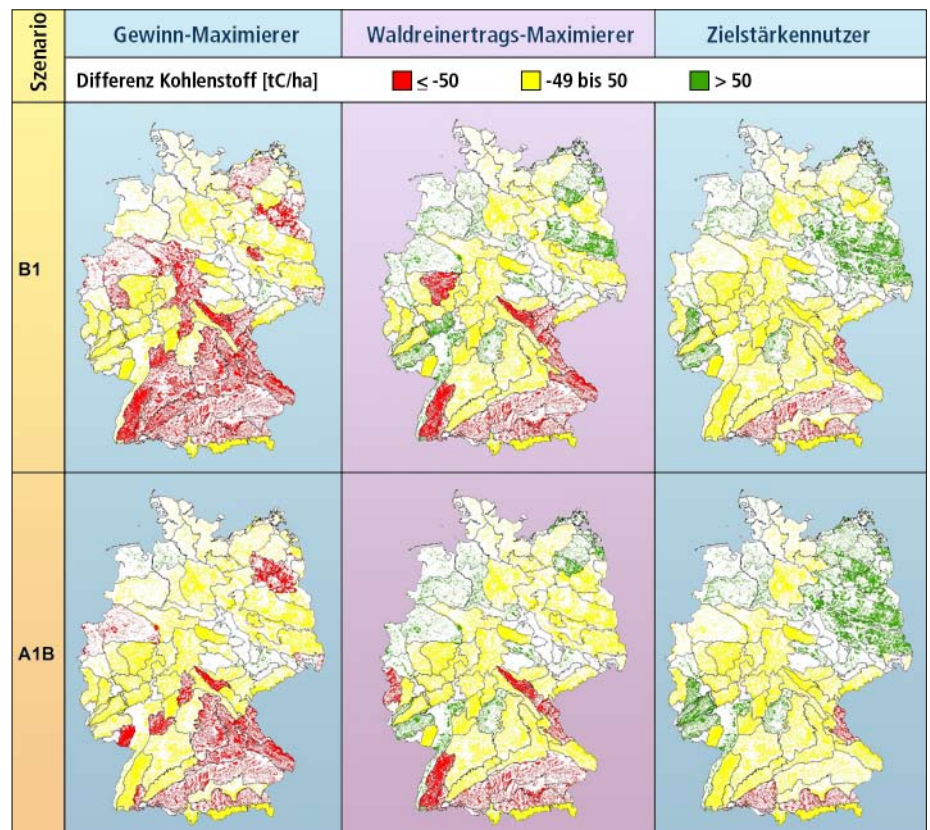
Abb. 2: Veränderung des Waldkohlenstoffspeichers [tC/ha] zwischen 2000 und 2100 nach Betriebsstypen und Szenarien (rot = Speicherabnahme, grün = Speicherzunahme, gelb = keine Speicheränderung)
