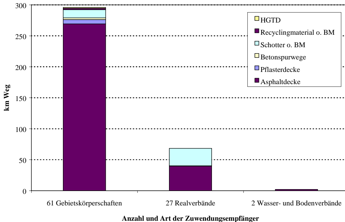
Abbildung r4: Anteile der Bauweisen an der gesamten Wegelänge, aufgeteilt nach Art der Zuwendungsempfänger
