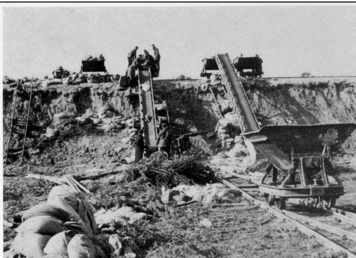
Abb. 9.5 Deichschäden nach der Sturmflut vom 16./17. Februar 1962 in der Gebietskulisse: II. Oldenburgisches Deichband hier: Augustgroden, ad-hoc Sicherungsarbeiten unmittelbar nach der Sturmflut
