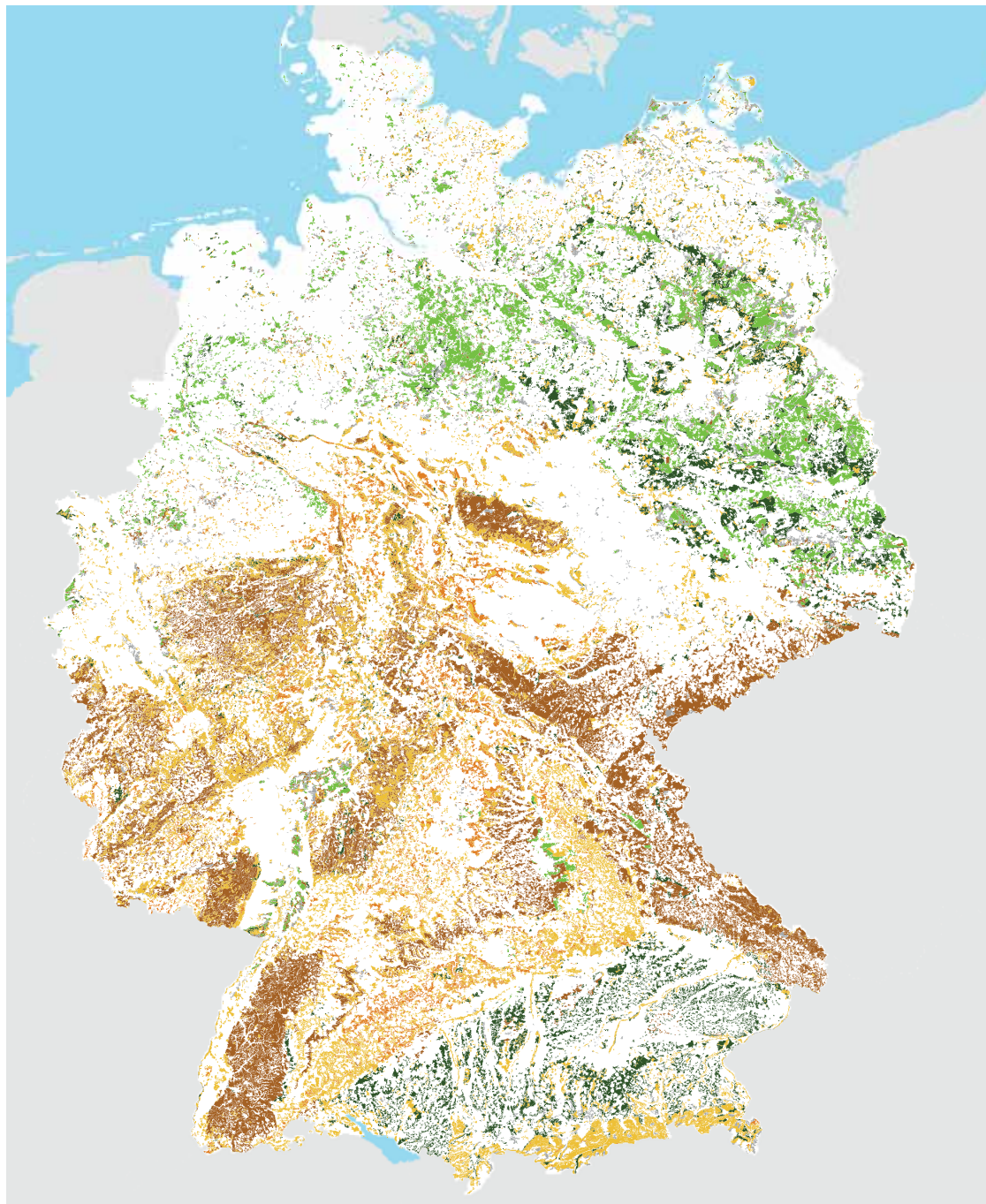
Karte 1: Regionale Verteilung der jährlichen Änderungsraten der organischen Kohlenstoffvorräte (t ha -1 ) in der organischen Auflage zwischen 1990 und 2006 unter Wald in Deutschland
