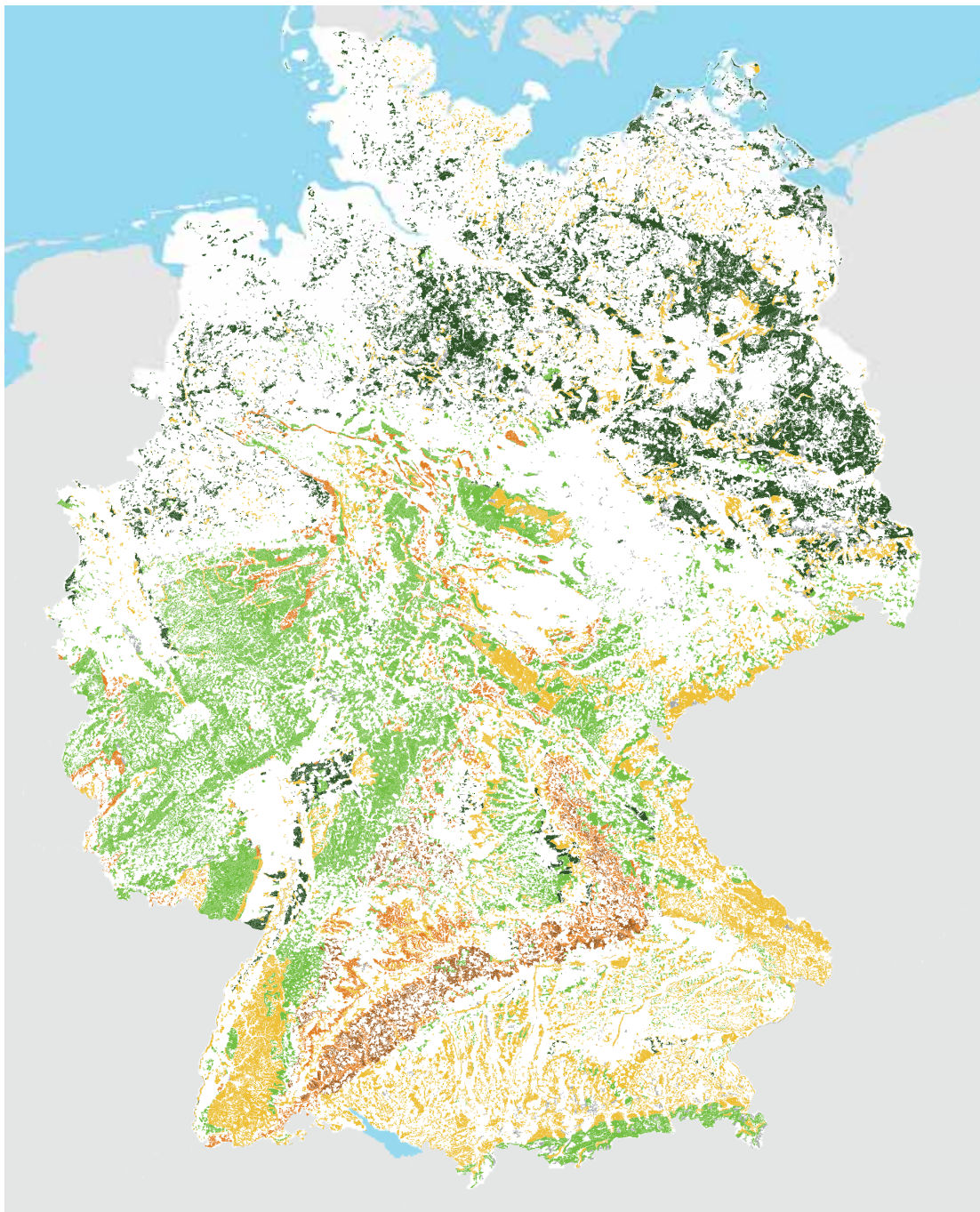
Karte 2: Regionale Verteilung der jährlichen Änderungs-raten der organischen Kohlstoffvorräte ( t\ ha^{-1} ) im Mineralboden (in 0 bis 30 cm Bodentiefe) zwischen 1990 und 2006 unter Wald in Deutschland
