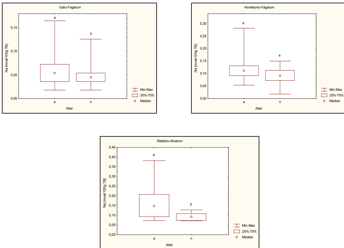
Abb. 20: Unterschiede der Natriumgehalte in Abhängigkeit vom Standortalter (U-Test).
