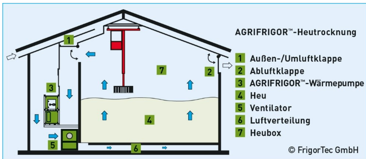
Bild 1: Das Agrifrigor-Verfahren am Beispiel einer Heutrocknung (Werkbild FrigorTec GmbH)
