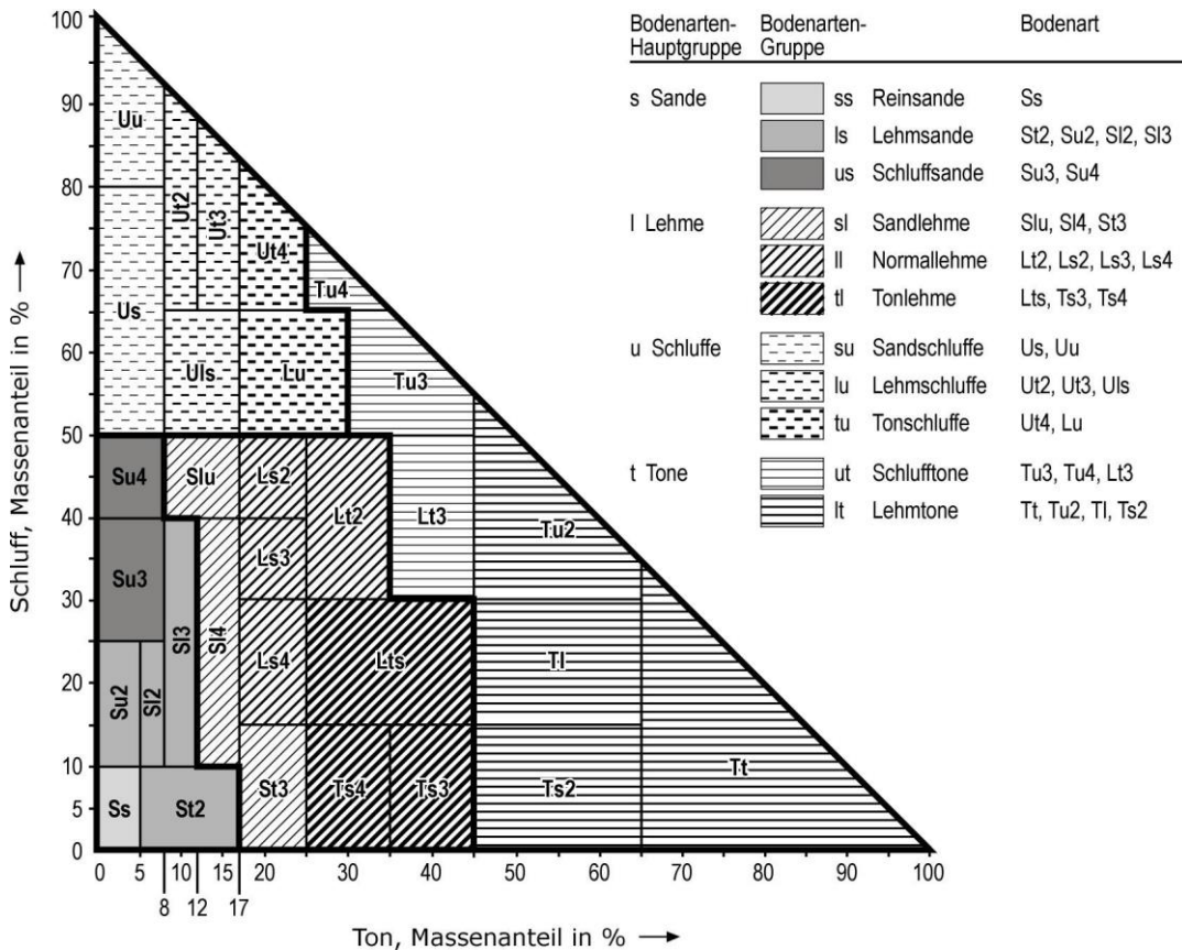
Abbildung IV-2: Diagramm zur Klassifikation der Feinbodenarten
