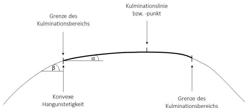
Abbildung III-1: Skizze zur Definition des Kulminationsbereichs
