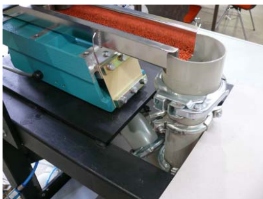
Abb. 5: Die Geschwindigkeit der Vibrationsrinne wird automatisch geregelt.
