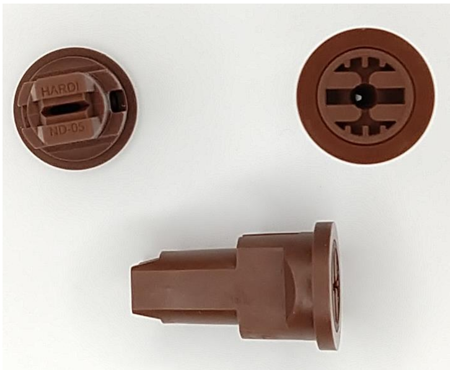
Flachstrahldüse HARDI NanoDrift ND 05 (Kunststoff, braun)
