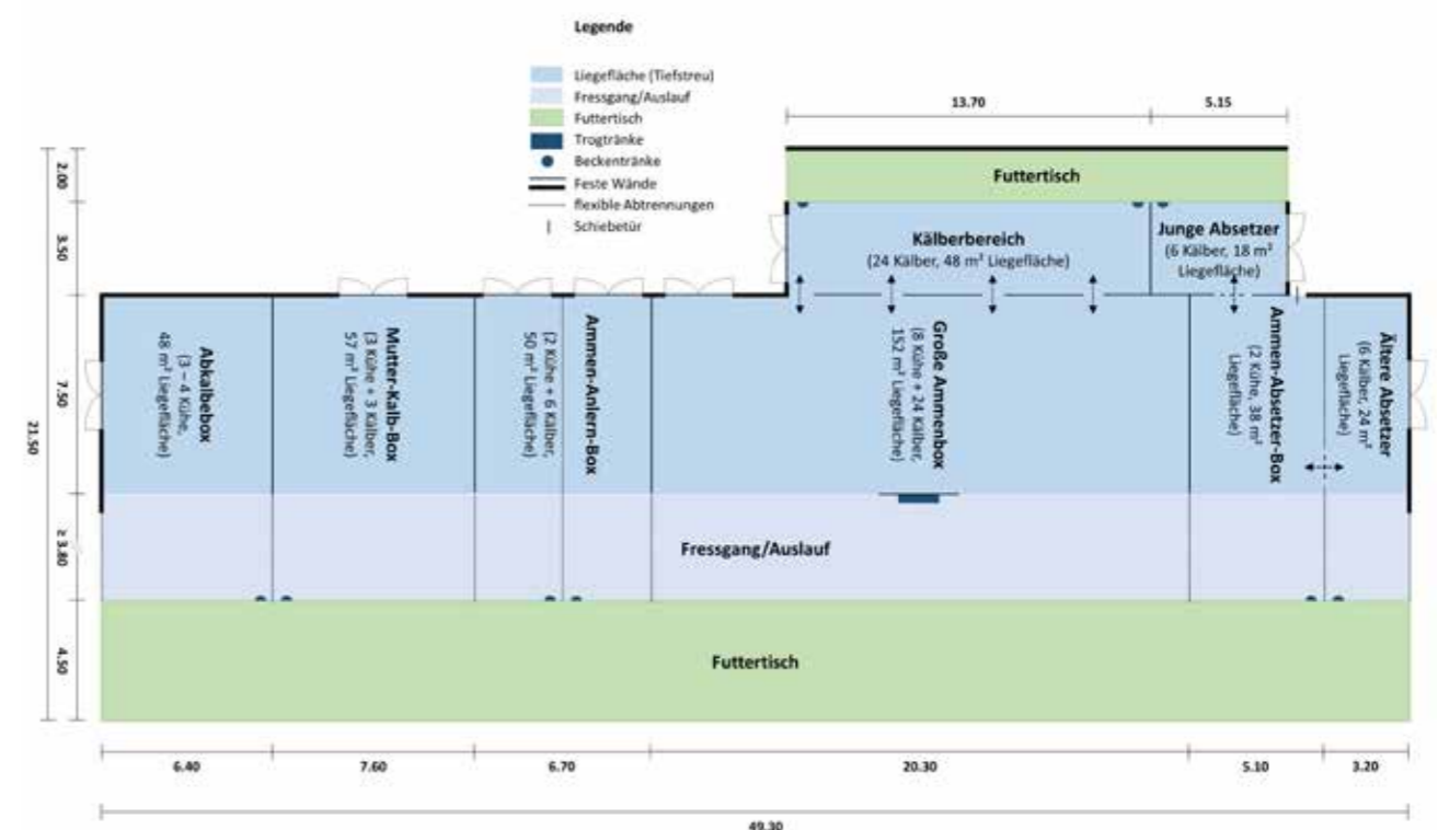
Exemplarischer Grundriss für einen Stall für eine Ammenaufzucht im mittelgroßen Betrieb
