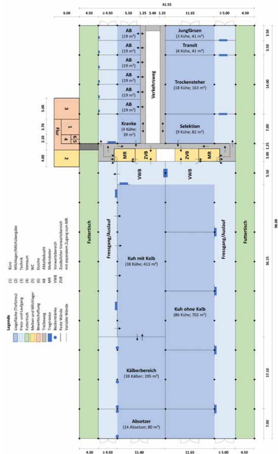
Exemplarischer Grundriss für einen Stall für eine muttergebundene Kälberaufzucht mit ganz-/ halbtäglichem Kuh-Kalbkontakt und Melkroboter
