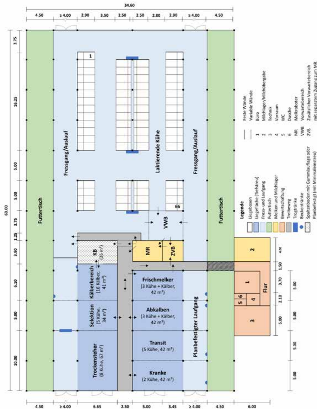
Exemplarischer Grundriss für einen Stall für eine muttergebundene Kälberaufzucht mit Kurzzeitkontakt und Melkroboter
