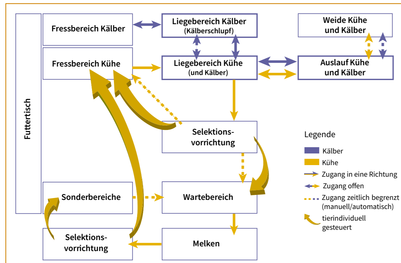
Funktionsschema für Verfahren mit Halb-/Ganztagskontakt, Kälberschlupf und selektivem Zugang zum Fress- bzw. Melkbereich
