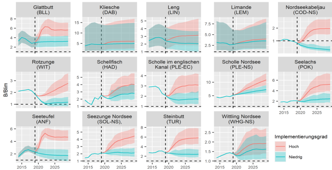
Abbildung 1: Laicherbestandbiomasse (B) in Relation zur Limitbiomasse (Blim) pro Bestand und Szenario. Median Werte (farbige Linien) und Unsicherheitsbereiche (schraffierte Flächen; 5% und 95% Perzentil) bei 100 Iterationen werden dargestellt. Der Start der Simulationen (2019) und die Referenzlinie B/Blim = 1.0 sind als gestrichelte Linien eingezeichnet. Szenarien unterscheiden sich im Grad der Implementierung der Anlandeverpflichtung ("Hoch" – strikte Implementierung: Flotten setzen die Fischerei aus, sobald die erste Quote ausgefischt ist; "Niedrig" – niedriger Implementierungsgrad: Fischerei stoppt nicht, wenn die erste Quote ausgefischt ist, sondern wird fortgesetzt, bis der Fischereiaufwand vom vorhergehenden Jahr erreicht wird). Quelle: Abgewandelt aus ProByFish Final Report (2021).
