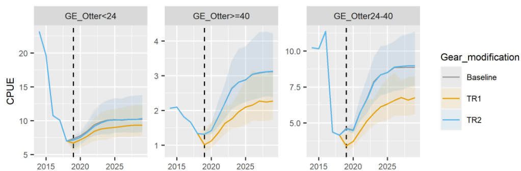
Abbildung 2: Fang pro Aufwandseinheit (CPUE) für deutsche Flottensegmente und Fanggerätemodifikationen. Median (bunte Linien) und Variation der Werte bei 100 Iterationen (schraffierte Flächen; 5% und 95% Perzentil). Das Anfangsjahr der Simulationen (2019) ist durch die gestrichelte Linie markiert. Die Baseline ohne weitere Modifikationen wird meist von der blauen Linie verdeckt. Im TR1 Szenario werden größere Maschenweiten von 140mm bei Scheerbrettnetzen (engl. Otter Trawls) im Vergleich zu Maschenweiten von 100mm bis 120mm im Baseline Szenario getestet. Im TR2 Szenario wird eine Trennung des Fanges mit Sortiergittern bei Scheerbrettnetzen mit Maschenweiten zwischen 70mm und 99mm simuliert. Quelle: Abgewandelt aus ProByFish Final Report (2021).
