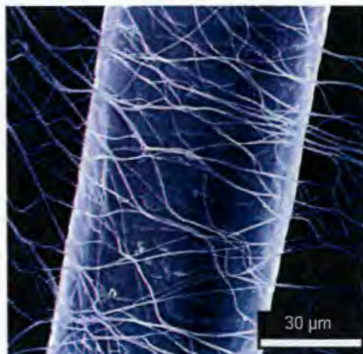
Abb.1 Elektrogessponnene Fasern im Größenvergleich mit einem menschlichen Haar
