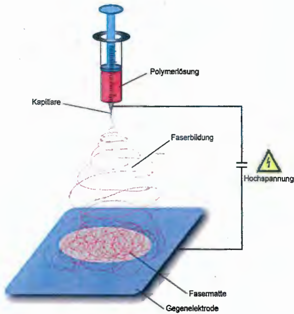
Abb.2 Schematische Darstellung Elektrospinsen
