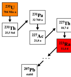
Abb. 3b: ^{235}\text{U} -Zerfallsreihe. Farblich dargestellt sind die im Grund- und Mineralwasser relevanten Radionuklide. Alle anderen spielen in der Regel aufgrund ihrer Löslichkeit und ihres Sorptionsverhaltens keine Rolle. Nach Hydroisotop (2007).
