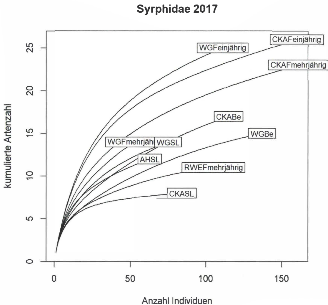
Abb. 4: Dargestellt ist die Anzahl der in 2017 auf den Flächen erfassten Schwebfliegenindividuen und -arten mit Hilfe sogenannter „accumulation curves“. Je steiler der Kurvenverlauf, desto mehr Arten wären bei weiteren Erfassungsterminen zu erwarten gewesen (WG = Wiesengut, CKA = Campus Klein Altendorf, AH/RWE = zusätzliche Fläche im weiteren Umfeld von Bonn).
