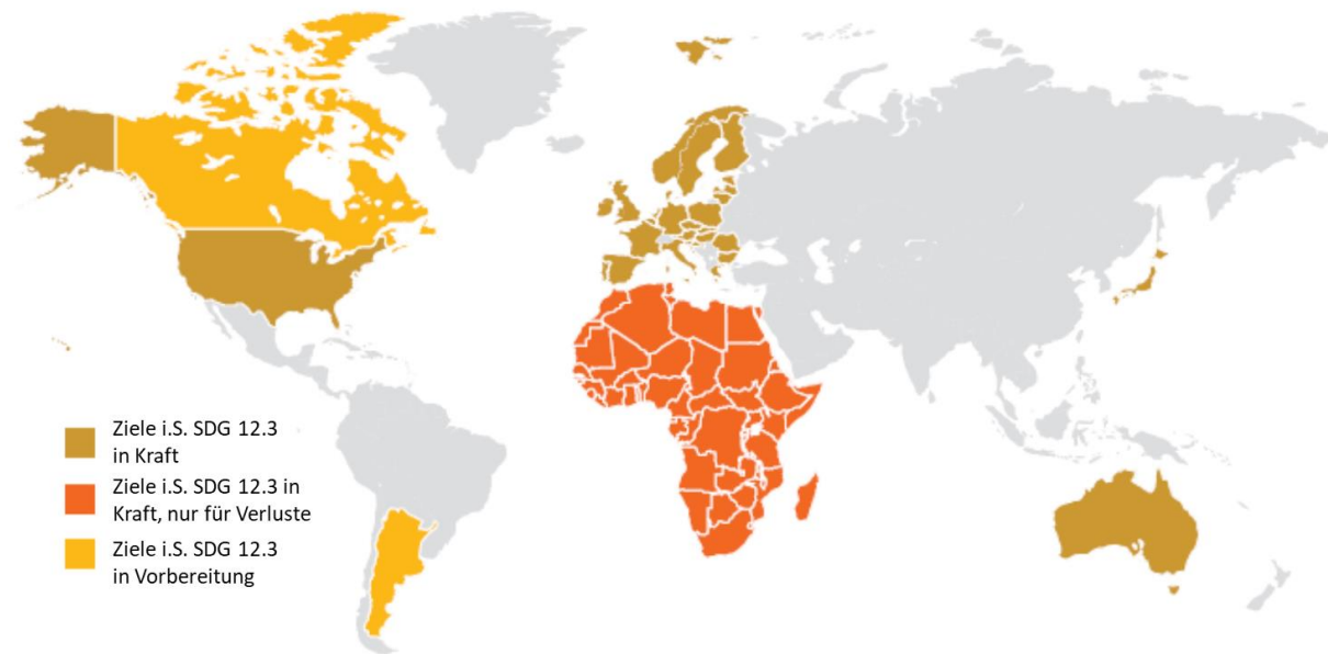
Abbildung 2: Vermeidungsziele für Lebensmittelverluste und -abfälle auf nationaler und regionaler Basis
