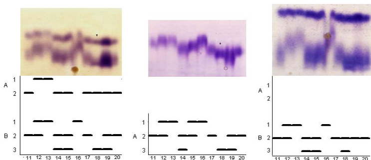
Abb. 1 Zymogramme und deren Interpretation (v.l.n.r) der Isoenzymssysteme Aconitase (ACO), Menadion-Reduktase (MNR) und Phosphogluco-Isomerase (PGI) der Individuen 11 bis 20 der Baldrianherkunft BLBP 45.
