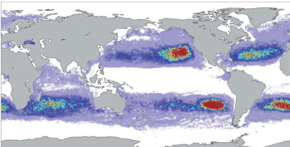
Abb. 1. Plastikmüllstrudel in den Ozeanen auf Basis der Simulation nach dem Vorhersagemodell von MAXIMENKO. Die roten Bereiche zeigen die Maximalkonzentrationen (DOHAN UND MAXIMENKO, 2010).
