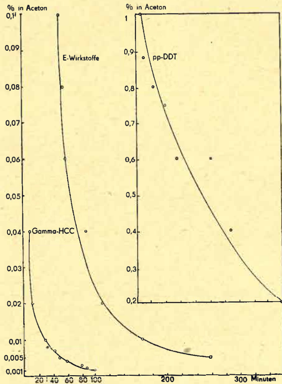
Abb. 1. Einwirkungszeit von Gamma-HCC, E-Wirkstoff und pp'-DDT auf Taufliegen bis zur Reglosigkeit in Abhängigkeit von der Wirkstoffmenge — gemessen an der Konzentration der Acetonlösung — auf Rundfilterplättchen.
