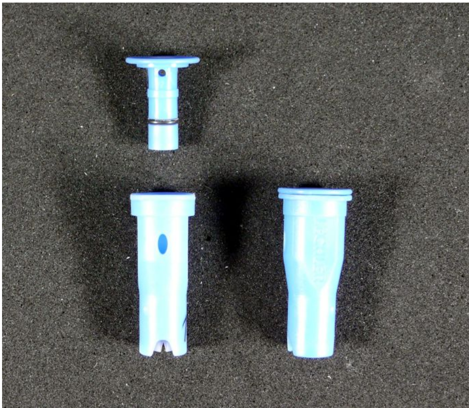
Flachstrahldüse ID-120-03 C (Keramik, kunststoffummantelt, blau)
