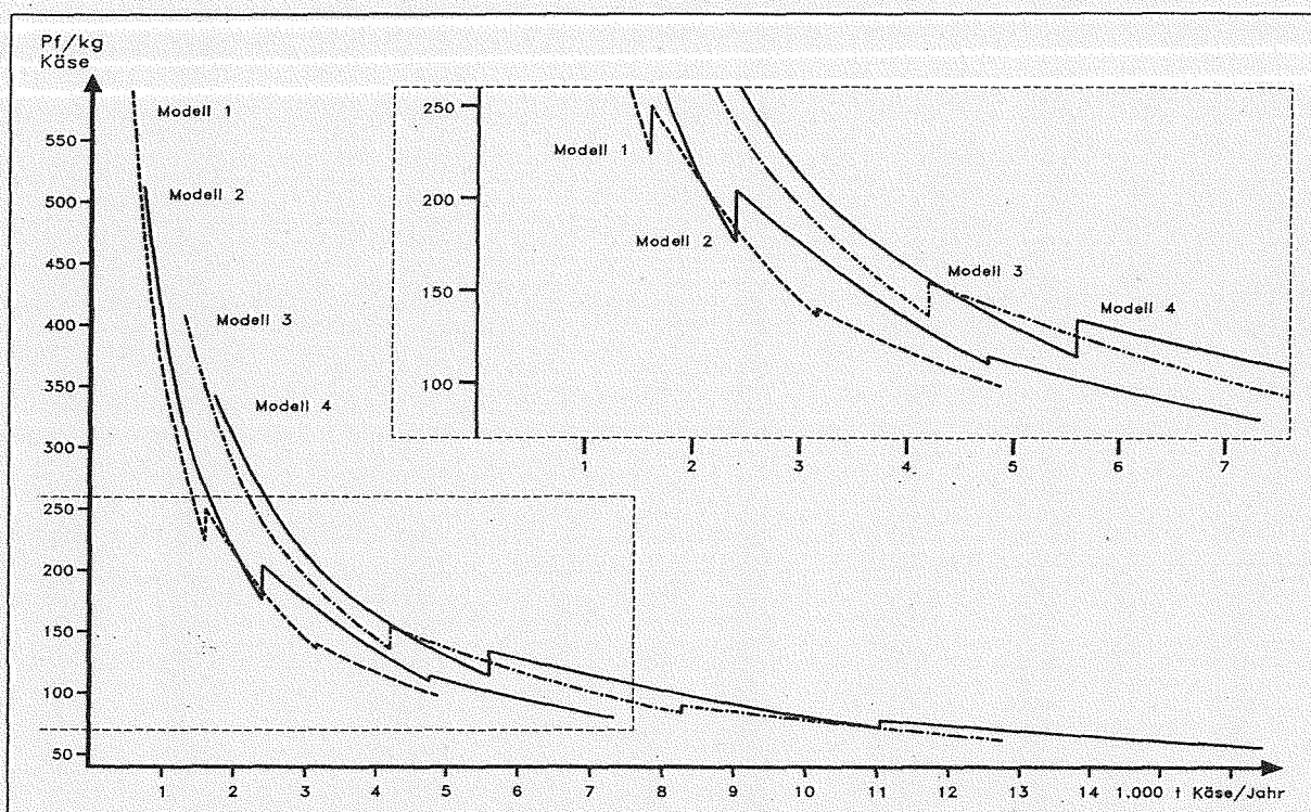
Abb. 7: Modellspezifische Einzelkosten der Abteilung Weichkäserei in Abhängigkeit von der Produktionsmenge (Pf/kg Abt.-Output)
