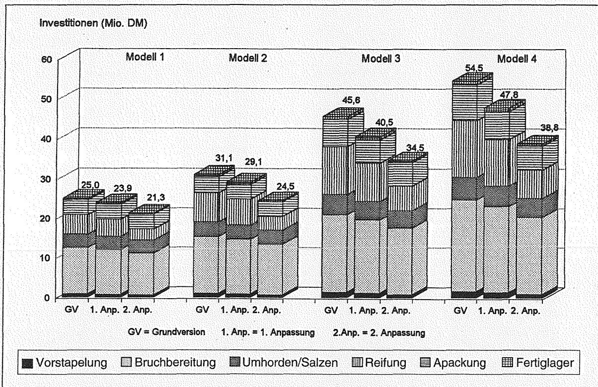
Abb. 1: Gesamtinvestitionen für die Abt. "Weichkäserei", gegliedert nach Unterabteilungen (Mio. DM) - Grundversion und Anpassungen
