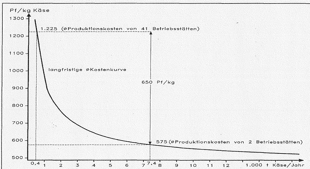
Abb. 20: Kostensenkungspotential durch Strukturveränderungen in Betriebsstätten <2.000 t Käse/Jahr
