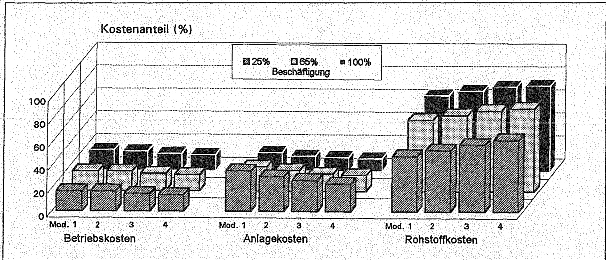
Abb. 11: Anteil der Kostenartengruppen an den Gesamtkosten der "Weichkäserei" (%)
