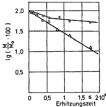
Abb. 5. Hitzeinaktivierung von Sojalipoxigenase in Anwesenheit von Lecithin ( 26,6 \mu\text{M} ) bei 60^\circ\text{C} und pH 7,0. ○ ohne Lecithin, △ mit Lecithin.
