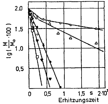
Abb. 4. Hitzeinaktivierung von Sojalipoxigenase in Anwesenheit von verschiedenen Fettsäuren (je 100 \mu\text{M} ) bei 60^\circ\text{C} und pH 7,0. ○ ohne Fettsäure, △ Stearinsäure, ● Palmitinsäure, + Myristinsäure, ▼ Linolsäure, □ Ölsäure.
