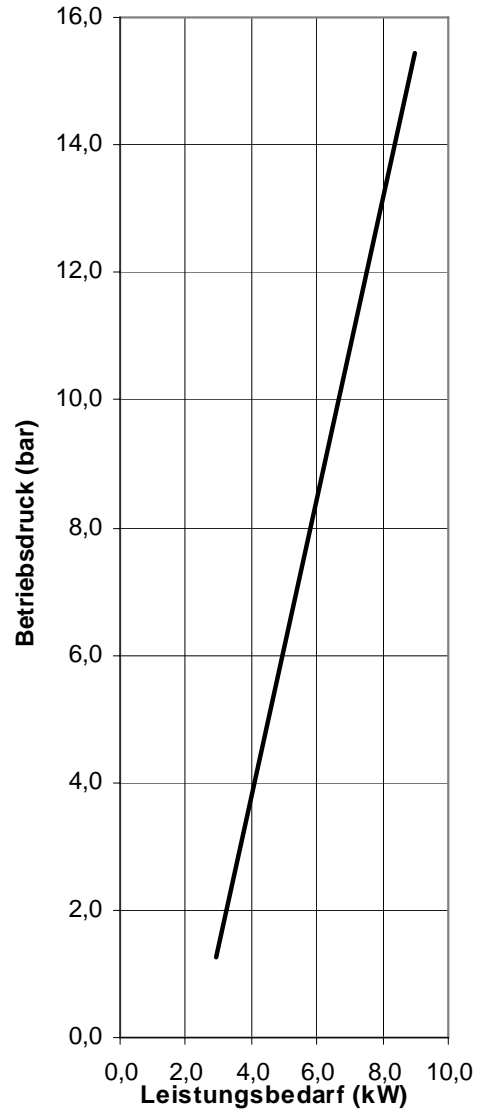
Bild 3: Leistungsbedarf altek P 260 bei 540 min -1
