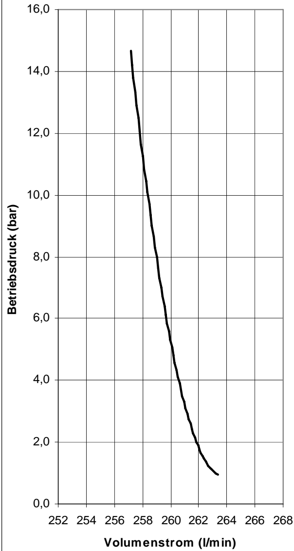
Bild 2: Pumpenvolumenstrom altek P 260 vor und nach Dauertest (200 h)
