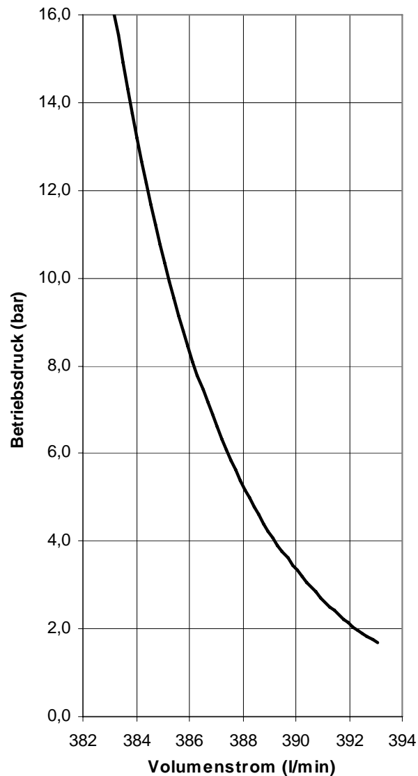
Bild 2: Pumpenvolumenstrom alte P 380 vor und nach Dauertest (200 h)
