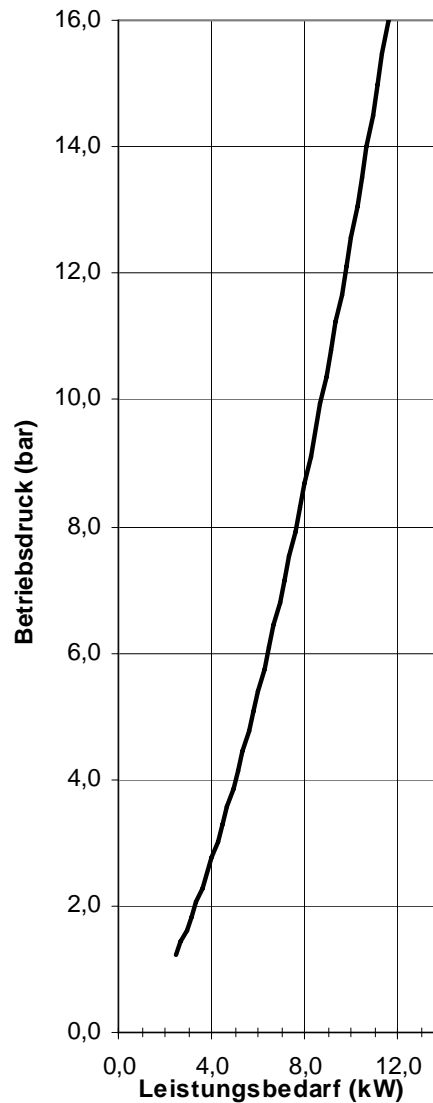
Bild 3: Leistungsbedarf alte P 380 bei 540 min -1
